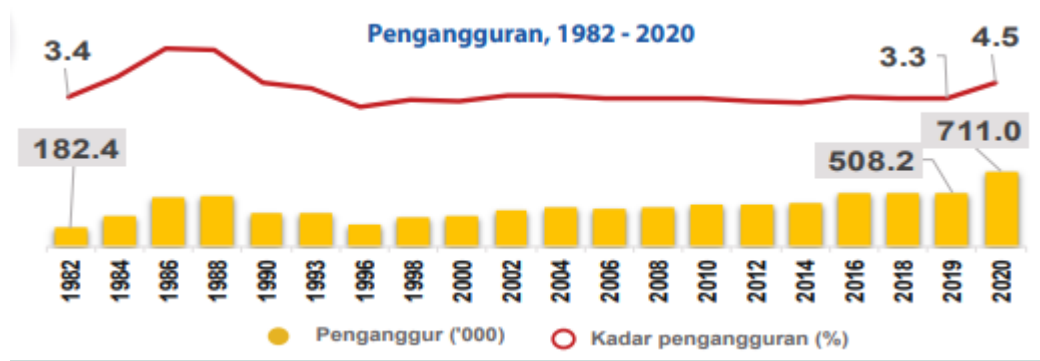
Rajah 1: Pengangguran 1982 – 2020
